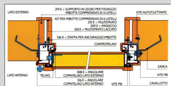
MONTAGGIO CON FINITURA LEGNO
