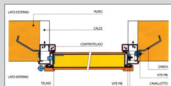
MONTAGGIO CON FINITURA INTONACO
