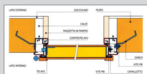
MONTAGGIO CON FINITURA MARMO
