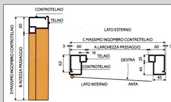
MISURE STANDARD PER TELAIO E CONTROTELAIO
